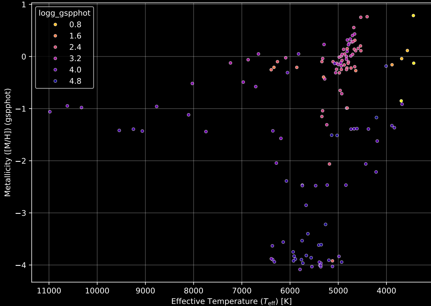
APOGEE DR17 Field: [000+05-O] Stellar Population Parameters (n= 142)
